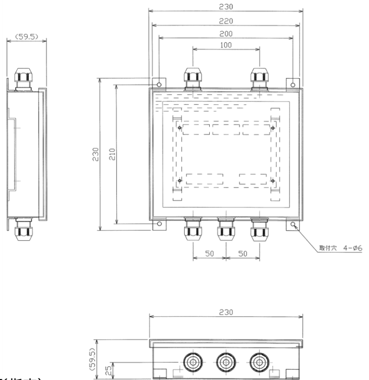
《外形寸法》
